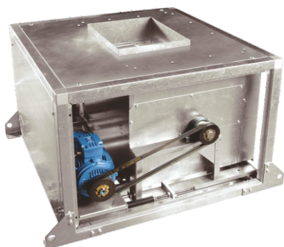
wersja z pionowym wyrzutem CVHT-V
