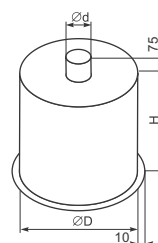
Skrzynka rozprężna okrągła z króćcem górnym
