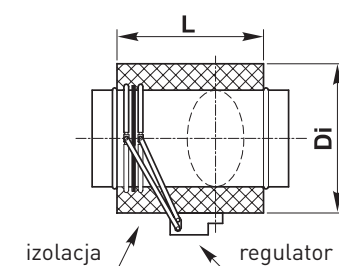
Rys. 3. regulator przepływu VAV typu: RVP-R, (z izolacją)
