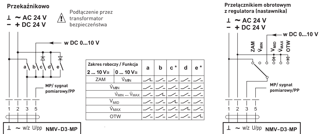
Schemat 1: Schemat podłączeń:
