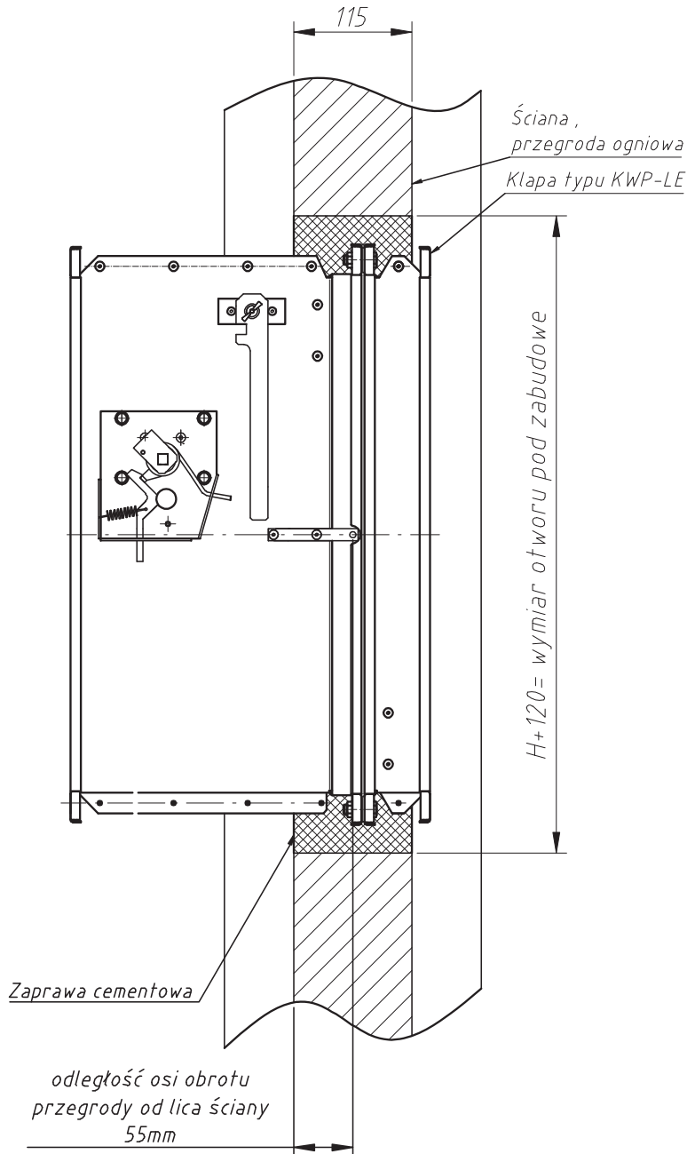
Rys. 4. Montaż klap odcinających typu KWP-L w przegrodach sztywnych
