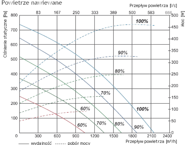
Powietrze nawiewane
