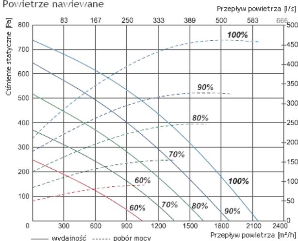
Powietrze nawiewane
