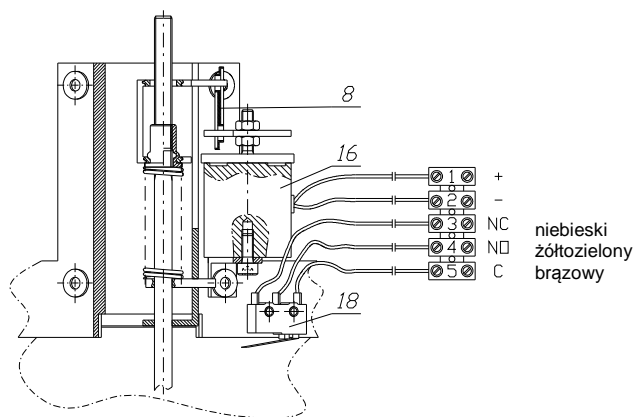
Rysunek 11. Podłączenie elementów elektrycznych w przeciwpożarowym zaworze odcinającym mcr ZIPP (8 - Wyzwalacz termiczny; 16 - Zwalniak elektromagnetyczny; 18 - Wyłącznik krańcowy WK1)
