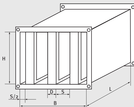
RYSUNEK ZŁOŻENIOWY
